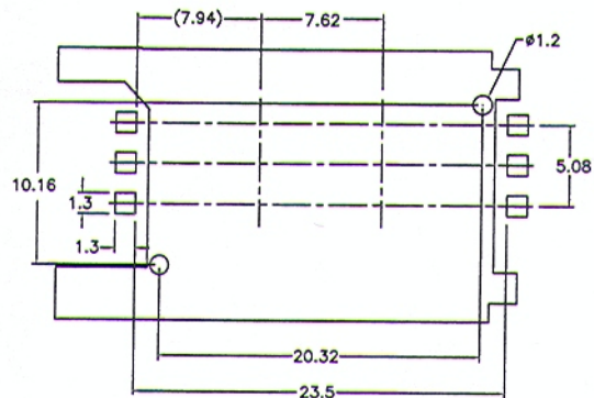
P.C.Board Layout
