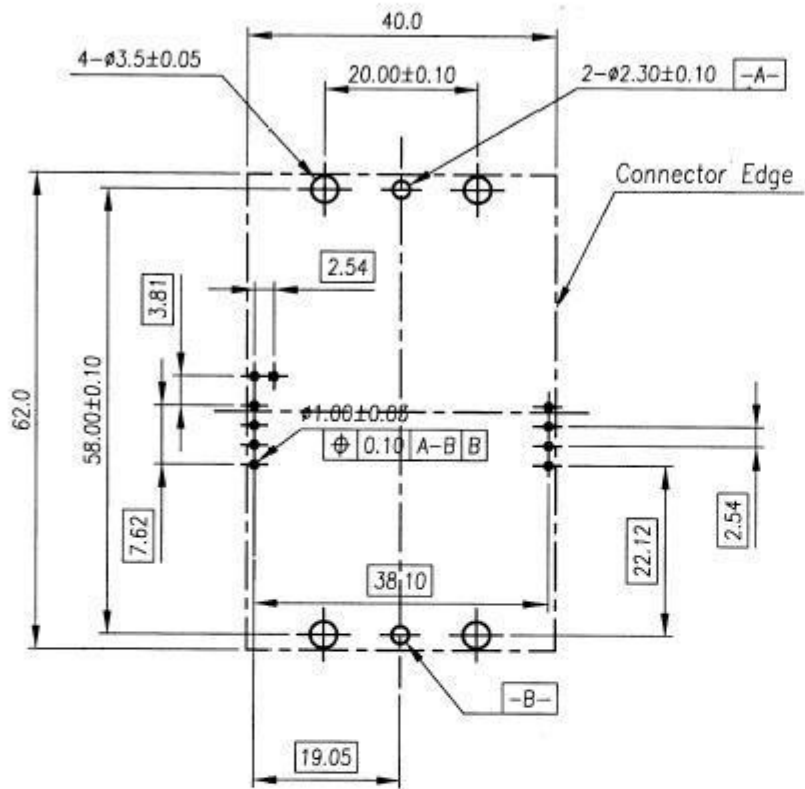
P.C.B. Layout
