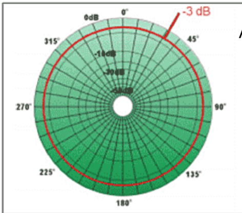
Charakterystyki promieniowania anteny w płaszczyźnie pionowej i poziomej
