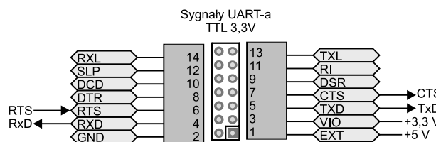
Rys. 5. Konfiguracja połączeń przy zasilaniu modułu z systemu, w którym został on zamontowany i współpracy z układami cyfrowymi zasilanymi napięciem 3,3 V
