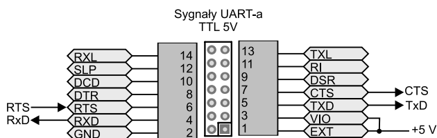
Rys. 4. Konfiguracja połączeń przy zasilaniu modułu z systemu, w którym został on zamontowany i współpracy z układami cyfrowymi zasilanymi napięciem 5 V (Uwaga! Styki 1 i 3 złącza CON2 można zewrzeć na płytce drukowanej – przewidziano miejsce na zworkę o rozmiarze 0805)
