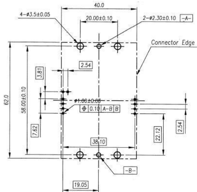
P.C.B. Layout
