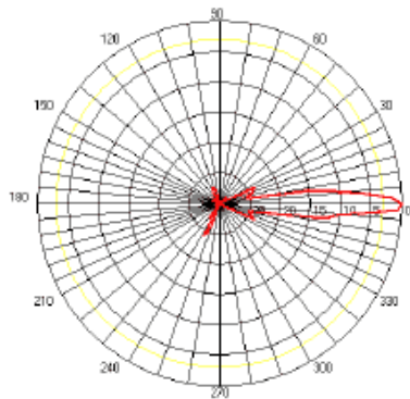
Charakterystyki kierunkowe anteny
